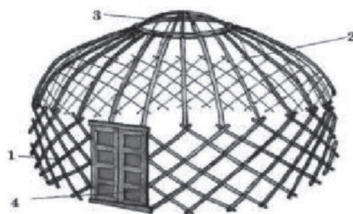
1 – кереге, 2 – уық, 3 – шаңырақ, 4 – сықырлауық
